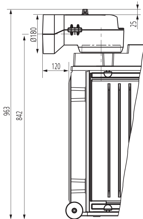
DIAMANT H13 mit waagrecht Heizgasstutzen Ø 180mm (Zubehör)
