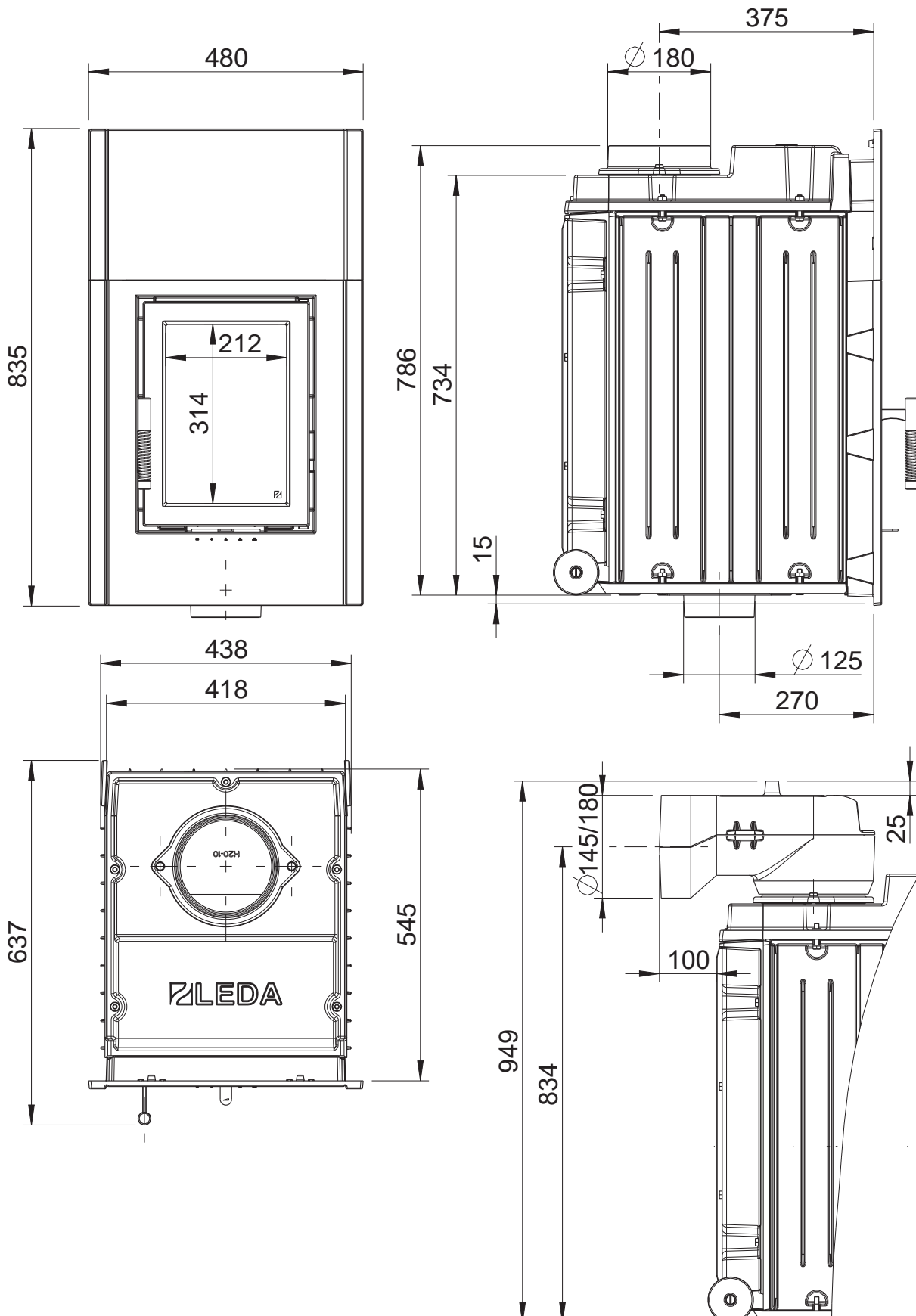
DIAMANT H20 mit waagrecht Heizgasstutzen \varnothing 180 mm (Zubehör)
