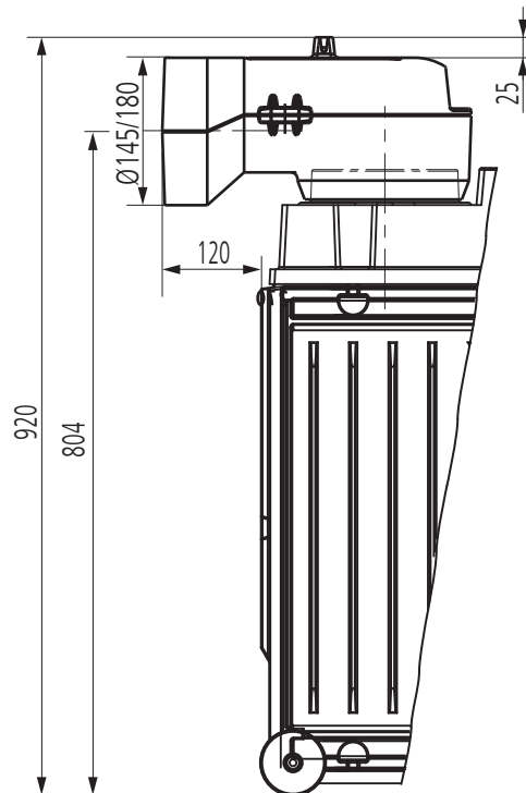
DIAMANT H10 mit waagrecht Heizgasstutzen Ø 180mm (Zubehör)
